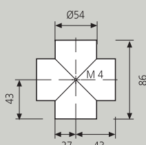
Conector en cruz Cross connector
