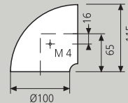
Empalme Coupler
