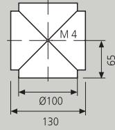
Arco 45° Bend 45°
