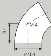
Arco 60° Bend 60°
