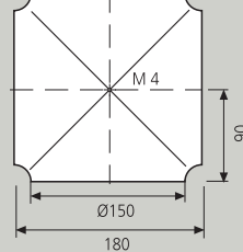
Conector en cruz Cross connector
