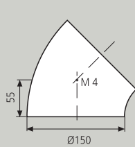
Arco 45° Bogen 45°
